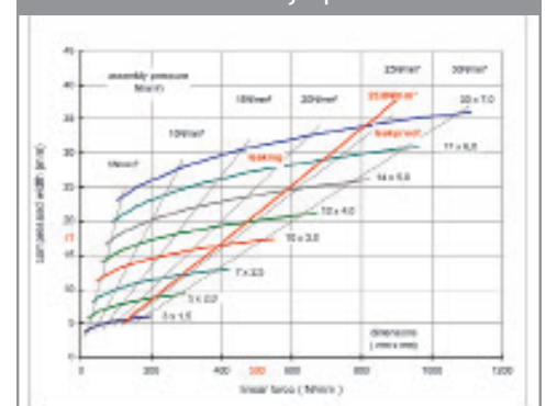
Deformación del ancho bajo apriete de TEADIT 24B
